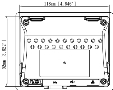
背视图
